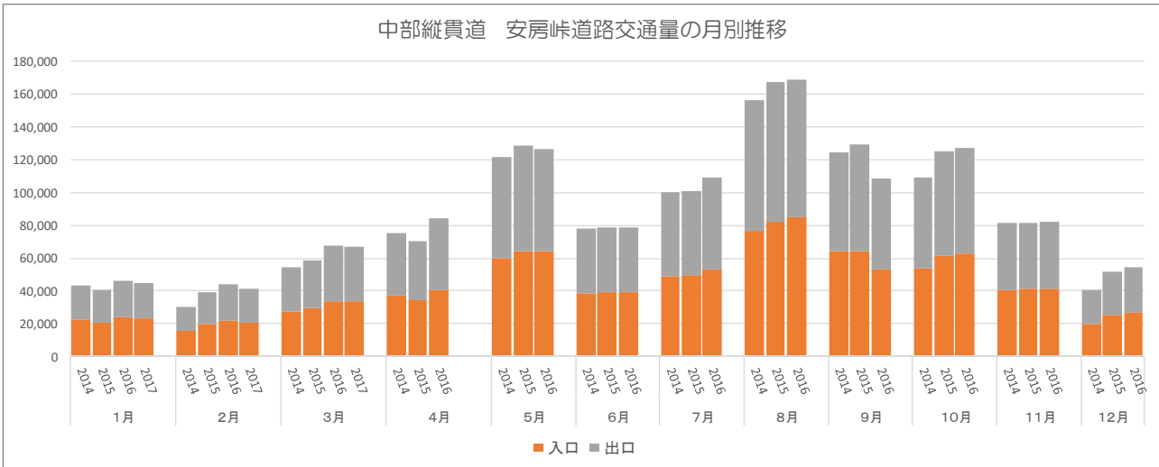
■中部縦貫道 安房峠道路交通量の月別推移 (資料: 中日本高速道路㈱ 松本保全サービスセンター安房峠道路営業所)
